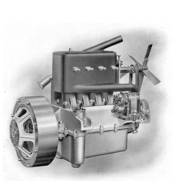
Moteur et Embrayage du châssis 12/14 HP
