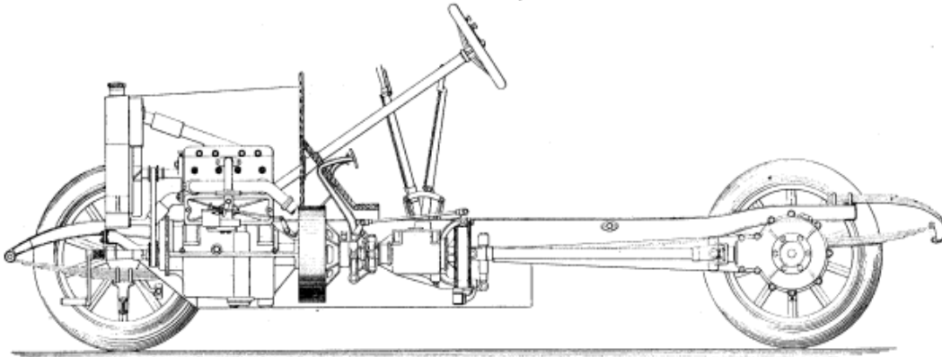
Exemple du châssis 12/14 HP
