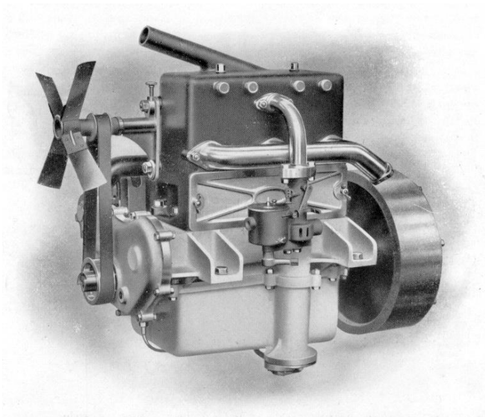
Moteur 12/14 HP côté du carburateur.
